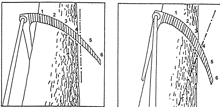
Abbildung 8: Winkelzählprobe - Zählfaktor 4 im Relaskopdurchblick
